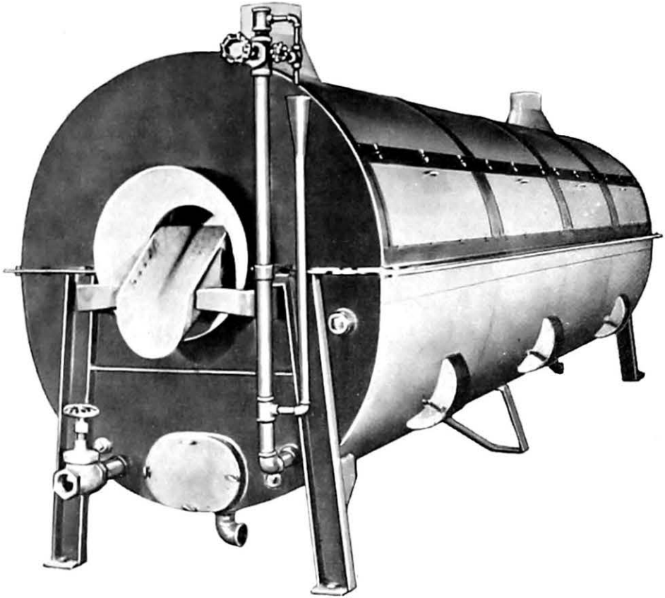
FIG. 34—Vegetable Blancher
