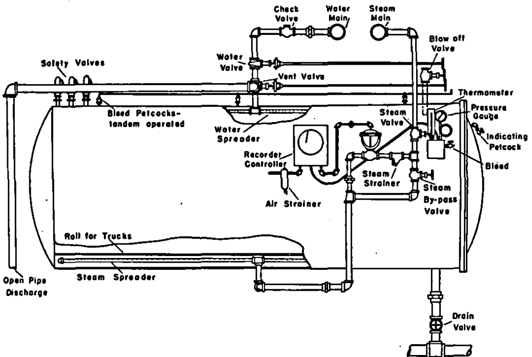
FIG. 31—Horizontal Retort
