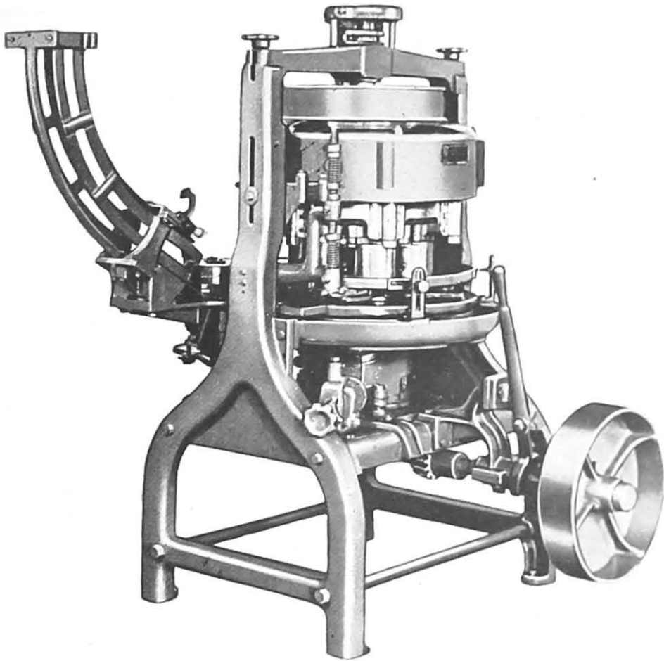
FIG. 38—Six-Pocket Plunger Filler
