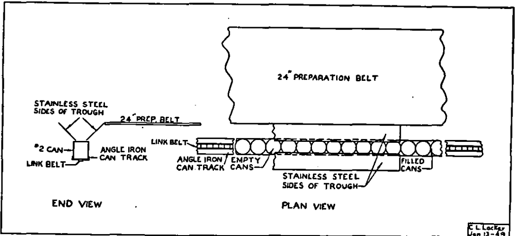
FIG. 27—Trough Filler
