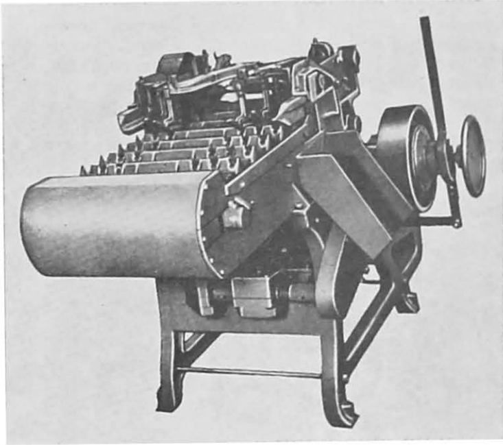
FIG. 35—Double Corn Husker
