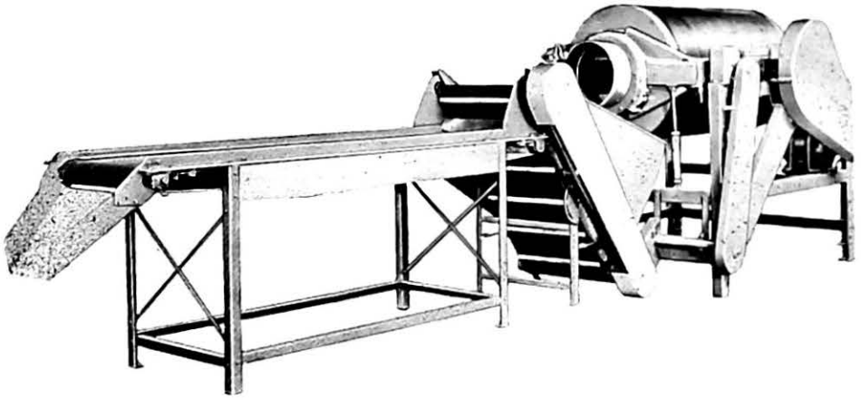
FIG. 32—Bean Snipper
