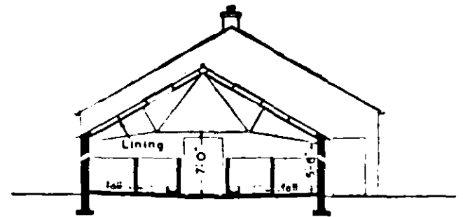
SECTION A-B
