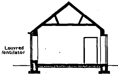
SECTION A-B.
