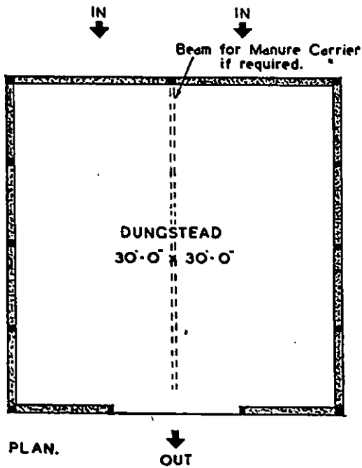
Fig. 36. Dungstead
