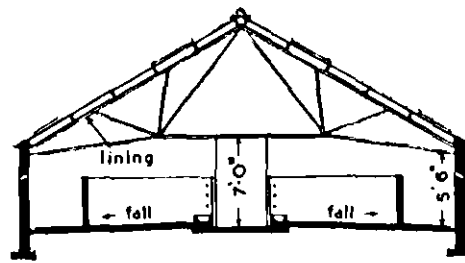
SECTION A-B
