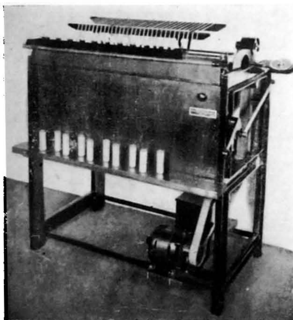
Fig. 37. Sizing reel.
