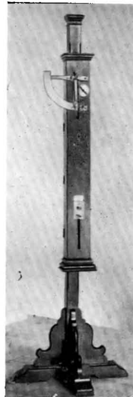
Fig. 41. Serimeter.
