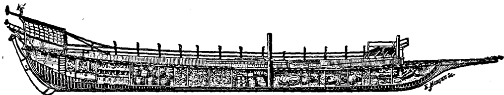
HOLD OF A GALLEY. ( Jurien de la Gravière. )
