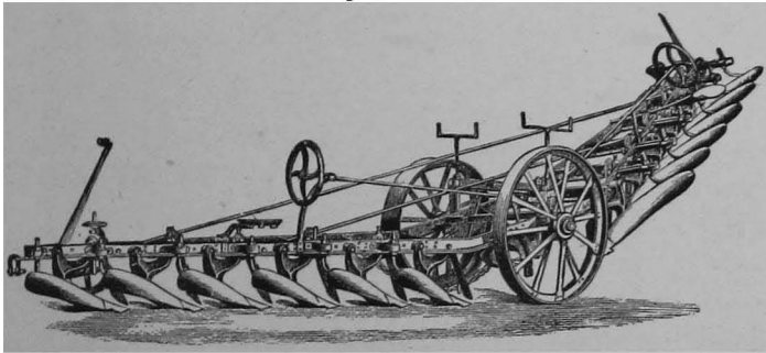
FIG. 18. GANG-PLOW.
