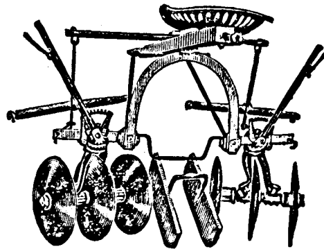
FIG. 32. DISC CULTIVATOR.
