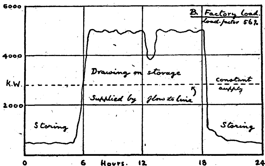
Fig. 17. Load factor diagram.
