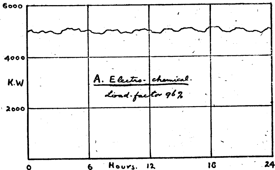
Fig. 16. Load factor diagram.
