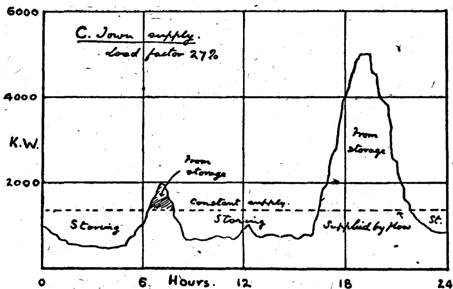
Fig. 18. Load factor diagram.
