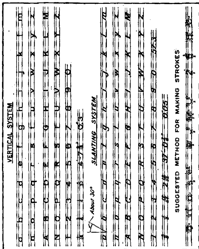
Fig. 26. — Lettering.
