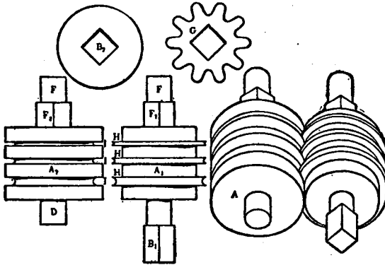
FIG. 14. PURNELL'S ROLLS
