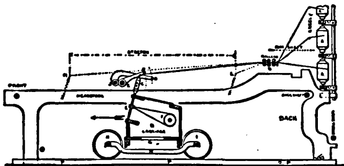
FIG. 4. CROMPTON'S MULE
