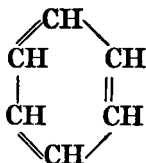
C_6H_6 , benzene.
