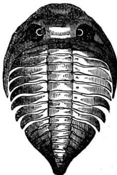
FIG. 10.—Trilobite.
