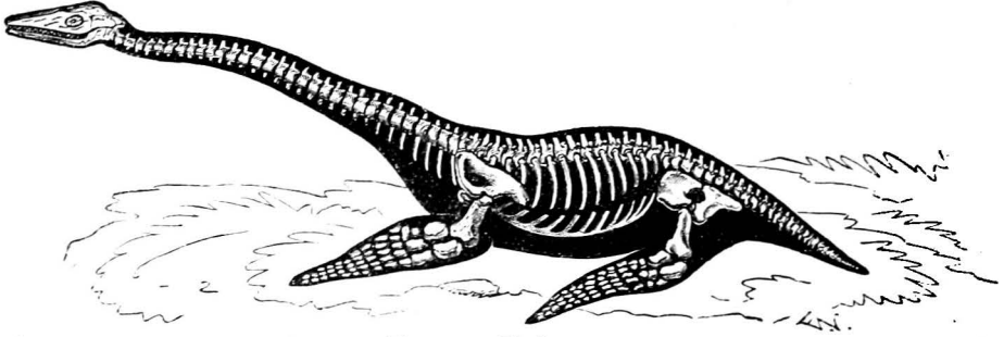
FIG. 15.—Plesiosaurus.
