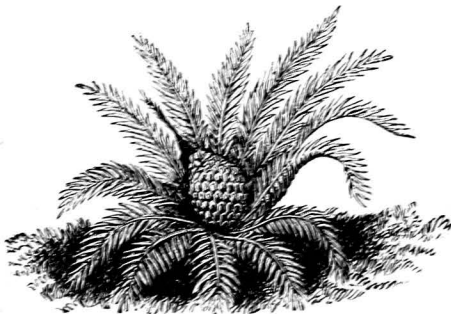
FIG. 32.—Cycad (Australia).
