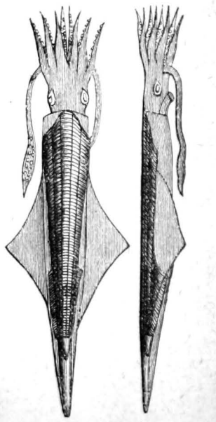
FIG. 14.—Belemnites.
