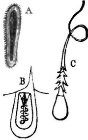
FIG. 39.—Hydra.
