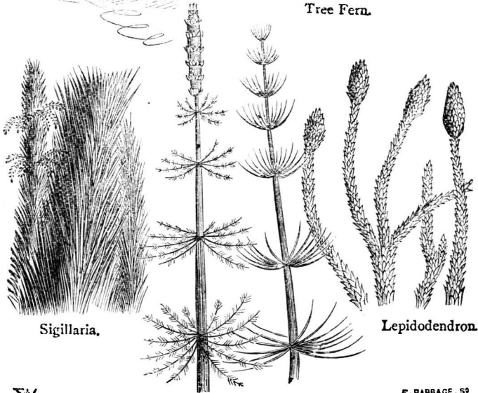
Calamite.
