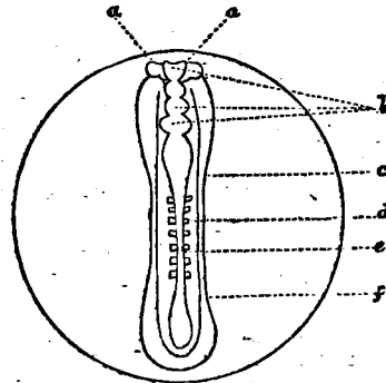
FIG. 69.—Embryo Stage.
