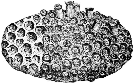
FIG. 42.—Coral.
