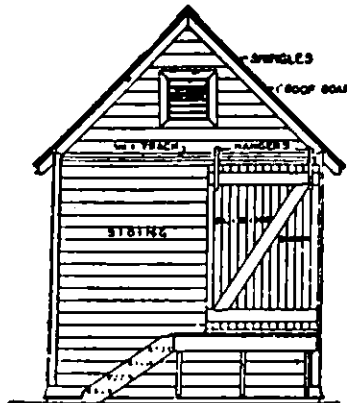
END ELEVATION
