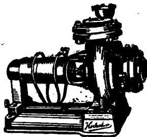
सेंट्रिफ्युगल पंप
