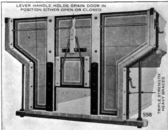
FIG. 10.—Dump end gate.
