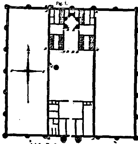
Fig. 1. Ground-plan of Palace at Mashita (after Triestram). a. Sculptured facade. b. c. d. e. f. g. h. i. j. k. l. m. n. o. p. q. r. s. t. u. v. w. x. y. z. aa. ab. ac. ad. ae. af. ag. ah. ai. aj. ak. al. am. an. ao. ap. aq. ar. as. at. au. av. aw. ax. ay. az. ba. bb. bc. bd. be. bf. bg. bh. bi. bj. bk. bl. bm. bn. bo. bp. bq. br. bs. bt. bu. bv. bw. bx. by. bz. ca. cb. cc. cd. ce. cf. cg. ch. ci. cj. ck. cl. cm. cn. co. cp. cq. cr. cs. ct. cu. cv. cw. cx. cy. cz. da. db. dc. dd. de. df. dg. dh. di. dj. dk. dl. dm. dn. do. dp. dq. dr. ds. dt. du. dv. dw. dx. dy. dz. ea. eb. ec. ed. ee. ef. eg. eh. ei. ej. ek. el. em. en. eo. ep. eq. er. es. et. eu. ev. ew. ex. ey. ez. fa. fb. fc. fd. fe. ff. fg. fh. fi. fj. fk. fl. fm. fn. fo. fp. fq. fr. fs. ft. fu. fv. fw. fx. fy. fz. ga. gb. gc. gd. ge. gf. gg. gh. gi. gj. gk. gl. gm. gn. go. gp. gq. gr. gs. gt. gu. gv. gw. gx. gy. gz. ha. hb. hc. hd. he. hf. hg. hh. hi. hj. hk. hl. hm. hn. ho. hp. hq. hr. hs. ht. hu. hv. hw. hx. hy. hz. ia. ib. ic. id. ie. if. ig. ih. ii. ij. ik. il. im. in. io. ip. iq. ir. is. it. iu. iv. iw. ix. iy. iz. ja. jb. jc. jd. je. jf. jg. jh. ji. jj. jk. jl. jm. jn. jo. jp. jq. jr. js. jt. ju. jv. jw. jx. jy. jz. ka. kb. kc. kd. ke. kf. kg. kh. ki. kj. kk. kl. km. kn. ko. kp. kq. kr. ks. kt. ku. kv. kw. kx. ky. kz. la. lb. lc. ld. le. lf. lg. lh. li. lj. lk. ll. lm. ln. lo. lp. lq. lr. ls. lt. lu. lv. lw. lx. ly. lz. ma. mb. mc. md. me. mf. mg. mh. mi. mj. mk. ml. mm. mn. mo. mp. mq. mr. ms. mt. mu. mv. mw. mx. my. mz. na. nb. nc. nd. ne. nf. ng. nh. ni. nj. nk. nl. nm. no. np. nq. nr. ns. nt. nu. nv. nw. nx. ny. nz. oa. ob. oc. od. oe. of. og. oh. oi. oj. ok. ol. om. on. oo. op. oq. or. os. ot. ou. ov. ow. ox. oy. oz. pa. pb. pc. pd. pe. pf. pg. ph. pi. pj. pk. pl. pm. pn. po. pp. pq. pr. ps. pt. pu. pv. pw. px. py. pz. qa. qb. qc. qd. qe. qf. qg. qh. qi. qj. qk. ql. qm. qn. qo. qp. qq. qr. qs. qt. qu. qv. qw. qx. qy. qz. ra. rb. rc. rd. re. rf. rg. rh. ri. rj. rk. rl. rm. rn. ro. rp. rq. rr. rs. rt. ru. rv. rw. rx. ry. rz. sa. sb. sc. sd. se. sf. sg. sh. si. sj. sk. sl. sm. sn. so. sp. sq. sr. ss. st. su. sv. sw. sx. sy. sz. ta. tb. tc. td. te. tf. tg. th. ti. tj. tk. tl. tm. tn. to. tp. tq. tr. ts. tt. tu. tv. tw. tx. ty. tz. ua. ub. uc. ud. ue. uf. ug. uh. ui. uj. uk. ul. um. un. uo. up. uq. ur. us. ut. uu. uv. uw. ux. uy. uz. va. vb. vc. vd. ve. vf. vg. vh. vi. vj. vk. vl. vm. vn. vo. vp. vq. vr. vs. vt. vu. vv. vw. vx. vy. vz. wa. wb. wc. wd. we. wf. wg. wh. wi. wj. wk. wl. wm. wn. wo. wp. wq. wr. ws. wt. wu. wv. ww. wx. wy. wz. xa. xb. xc. xd. xe. xf. xg. xh. xi. xj. xk. xl. xm. xn. xo. xp. xq. xr. xs. xt. xu. xv. xw. xx. xy. xz. ya. yb. yc. yd. ye. yf. yg. yh. yi. yj. yk. yl. ym. yn. yo. yp. yq. yr. ys. yt. yu. yv. yw. yx. yy. yz. za. zb. zc. zd. ze. zf. zg. zh. zi. zj. zk. zl. zm. zn. zo. zp. zq. zr. zs. zt. zu. zv. zw. zx. zy. zz.
